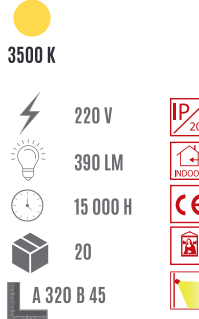
YDA 4006 / 6W 47.00 $ Led Yuvarlak Duvar Aplik • 180°
