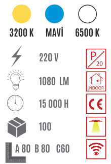
YMA 1045 / 1.5W Armatür Sensörlü (Radar)
